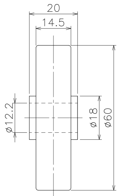
ホイール単品図
