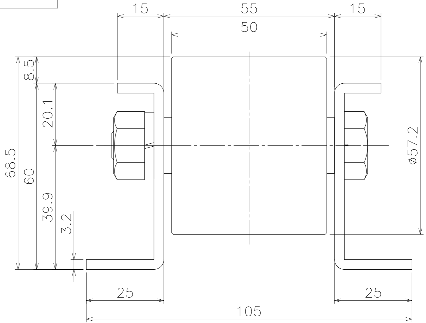
断面図
