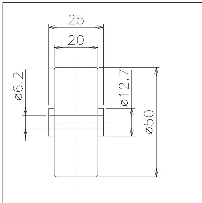
ホイル単品図
