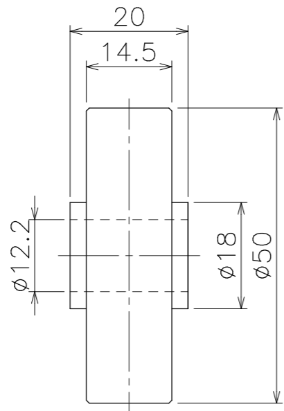
ホイール単品図
