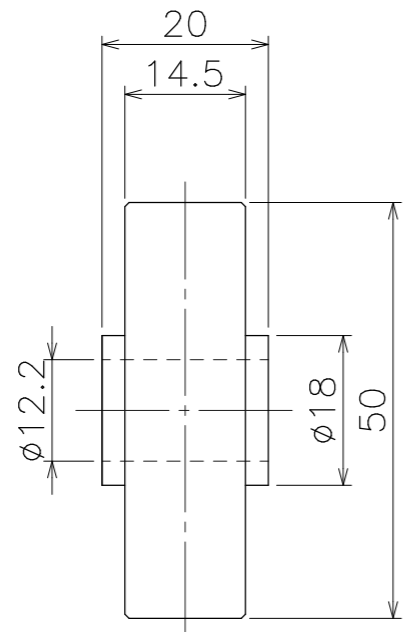
ホイール単品図
