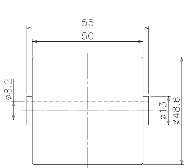
ホイール単品図
