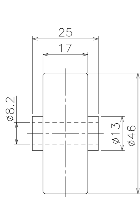
ホイール単品図
