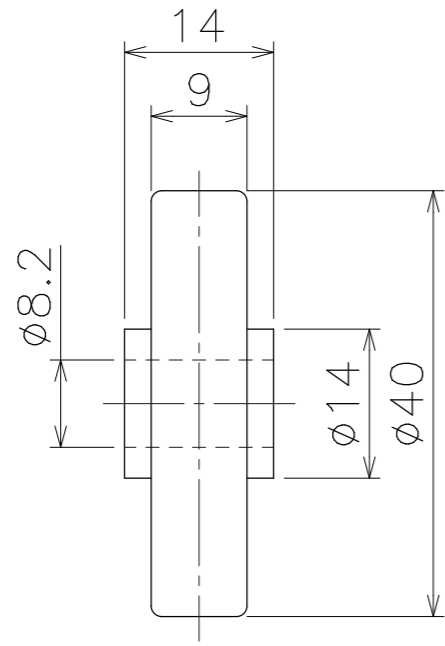
ホイール单品図
