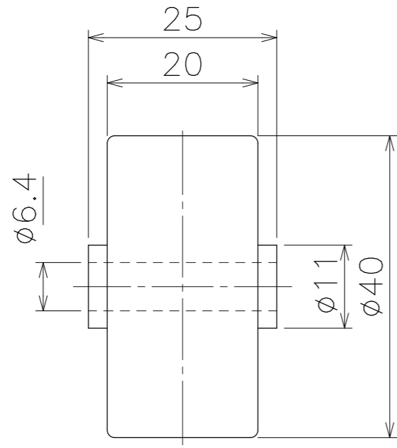
ホイール単品図
