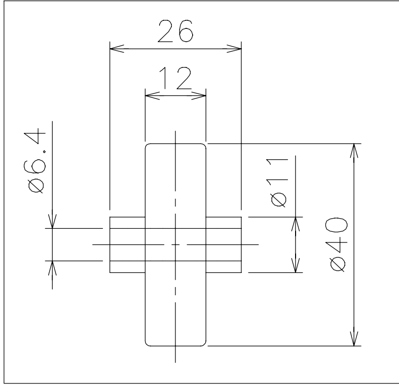
ホイール単品図
