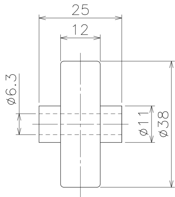
ホイール单品図
