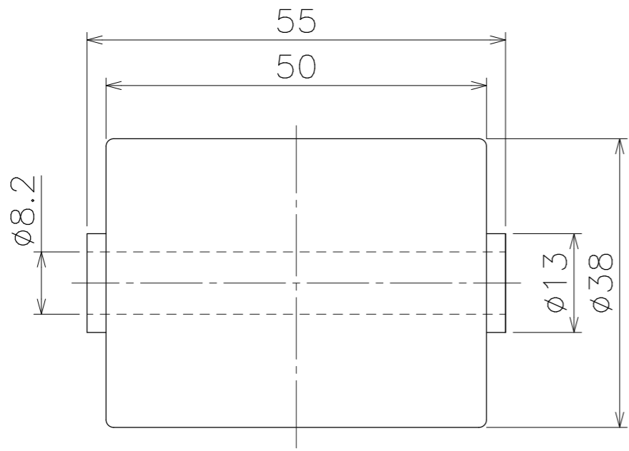
ホイール単品図
