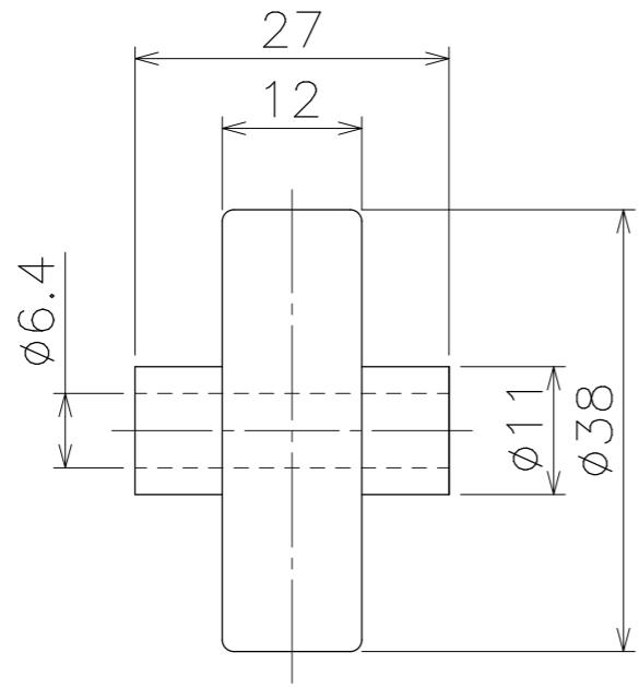
ホイール単品図
