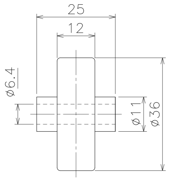
ホイール単品図
