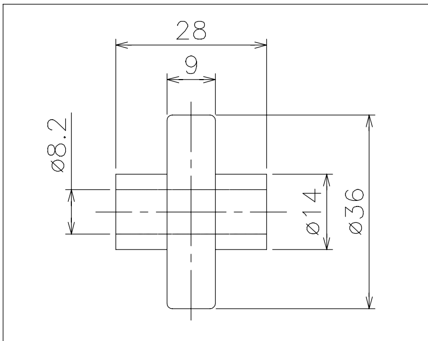
部品単一図
