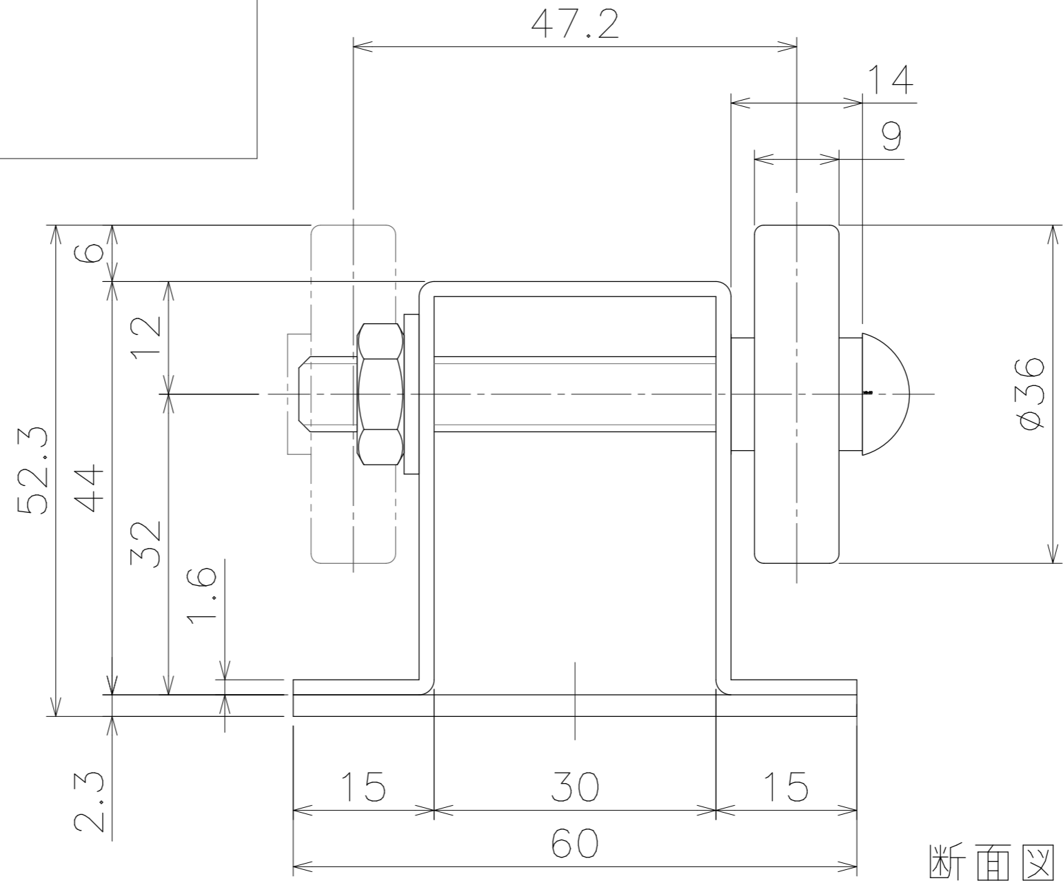
ホイール単品図
