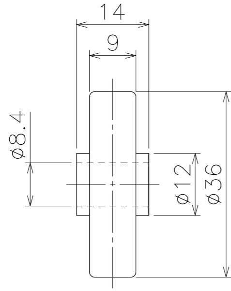
ホイール単品図
