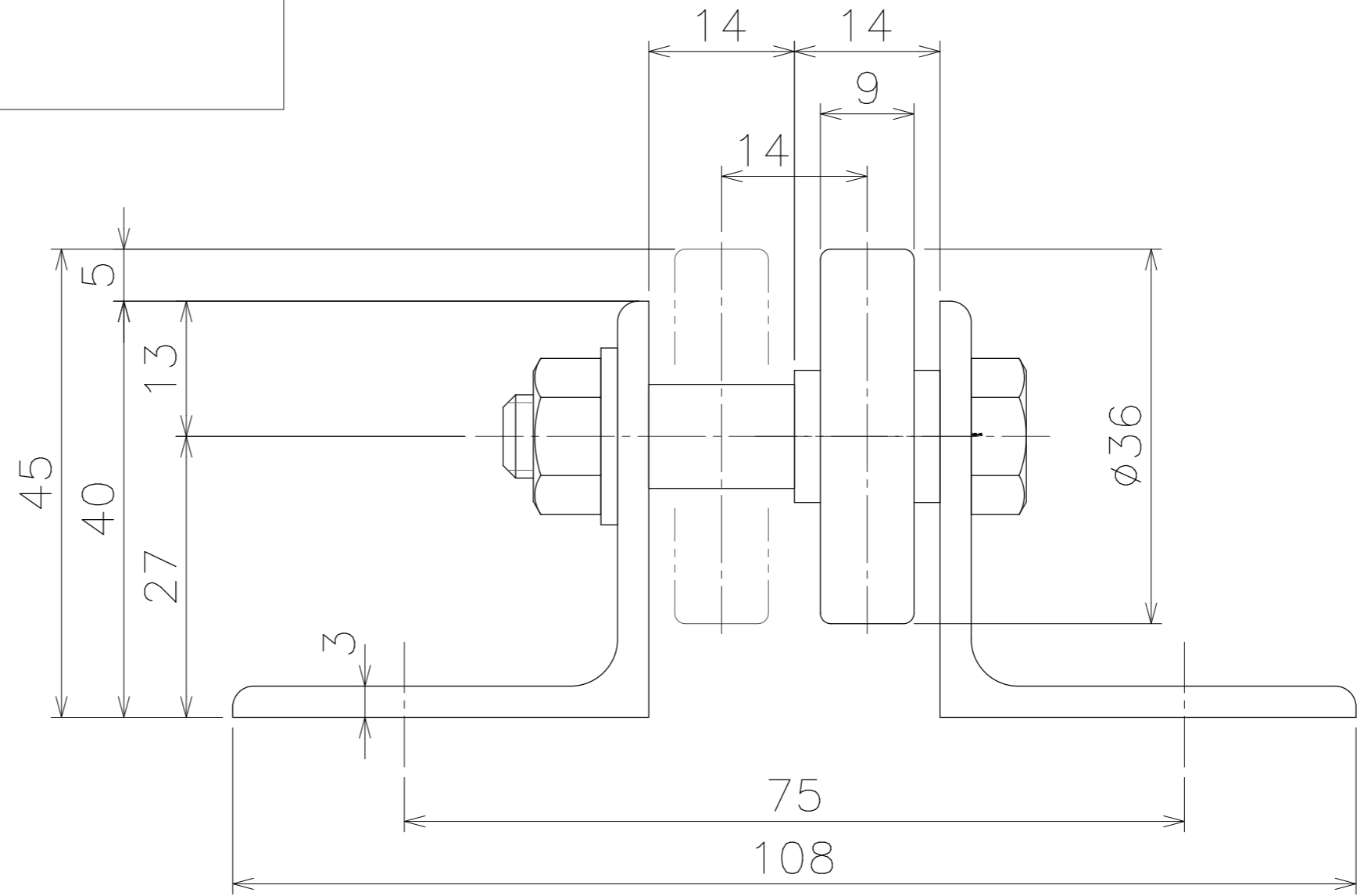
断面図
