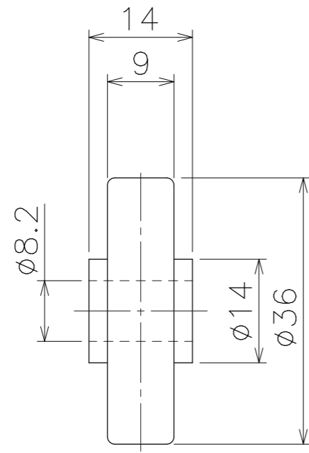
ホイール単品図
