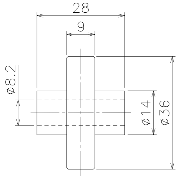
ホイール単品図
