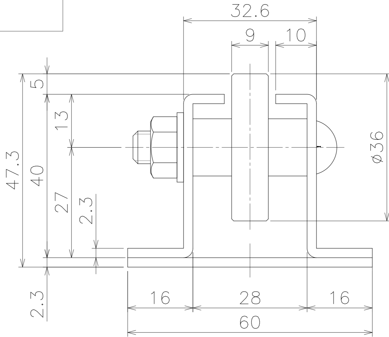
断面図
