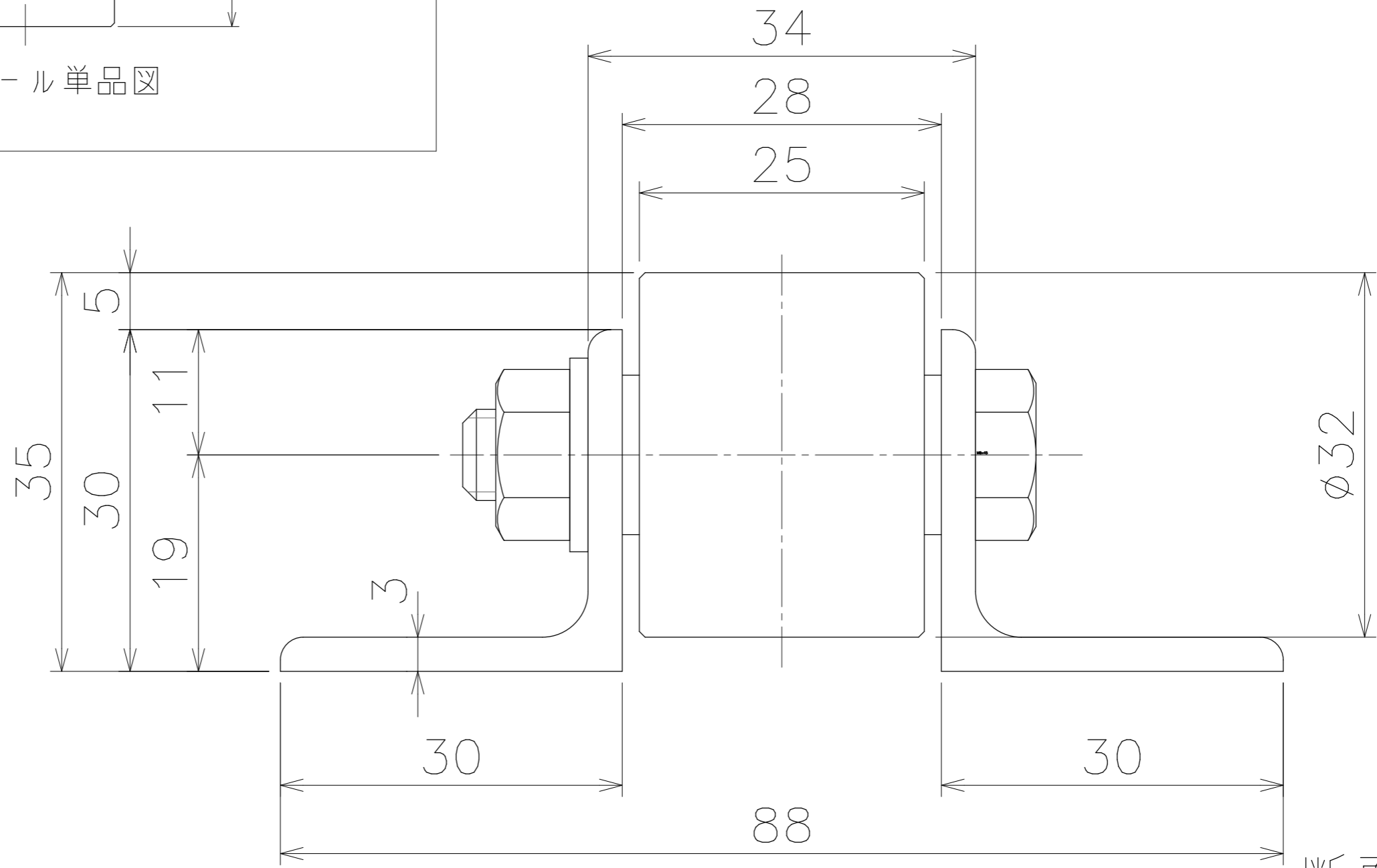
断面図
