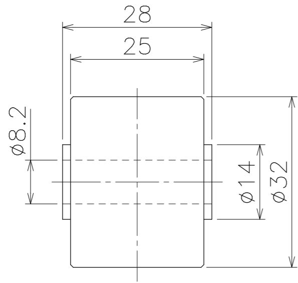
ホイール単品図
