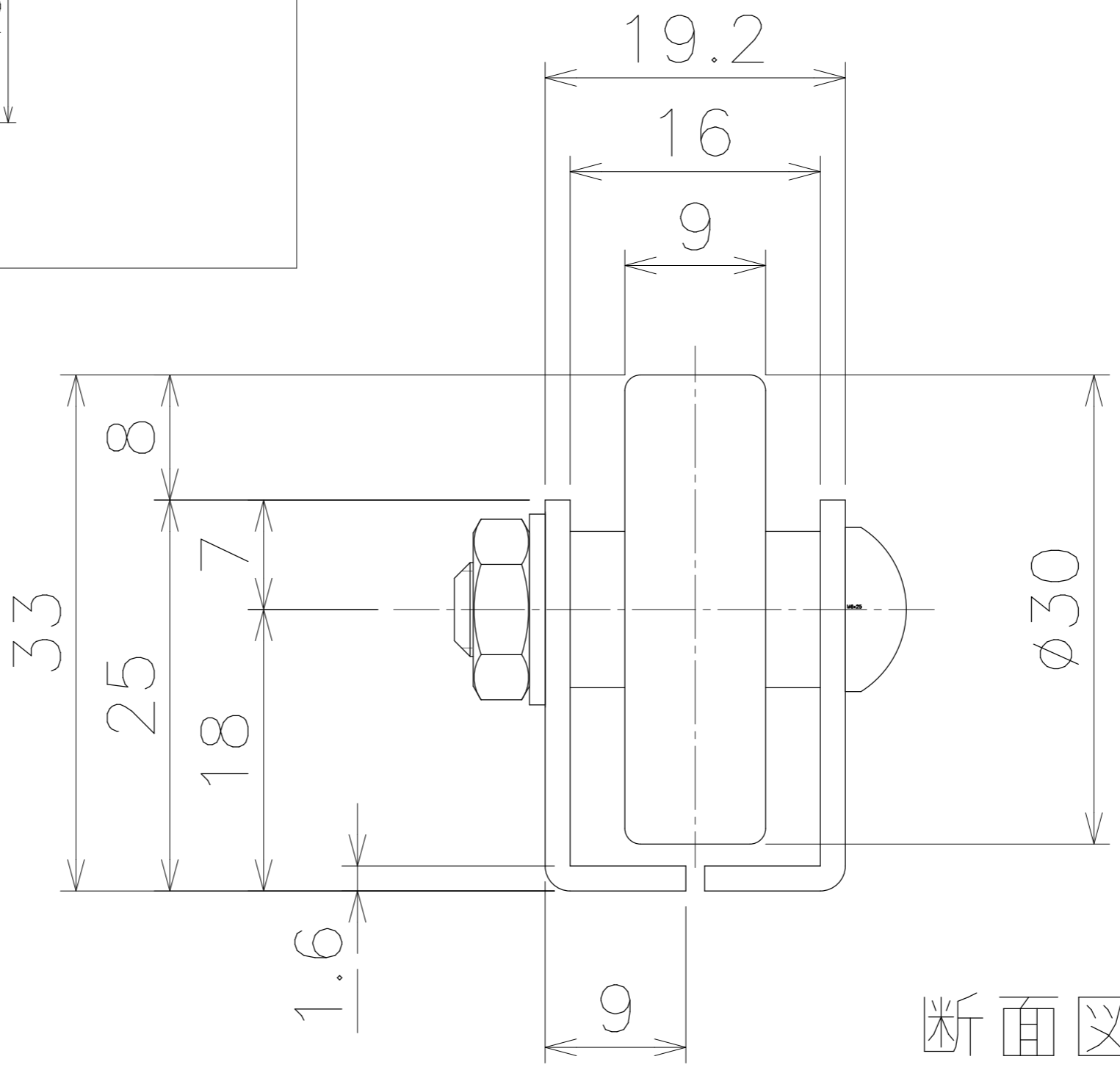
ホイール単品図
