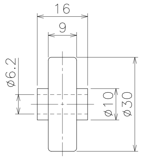
ホイール単品図
