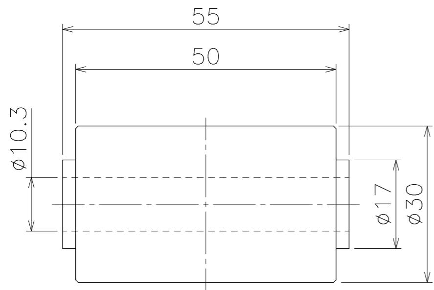
ホイール単品図
