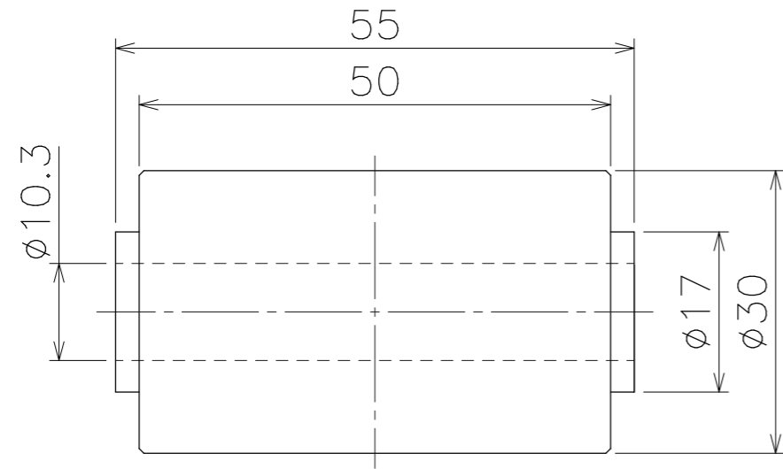
ホイール単品図
