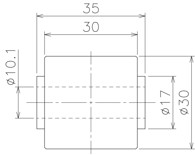
ホイール単品図
