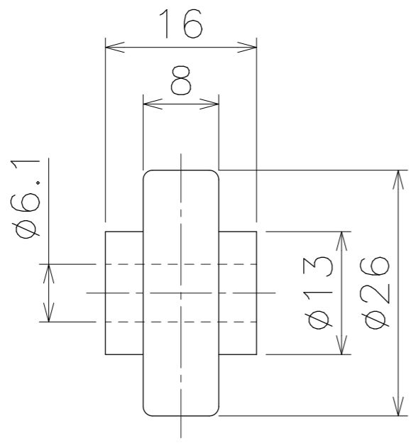
ホイール单品図
