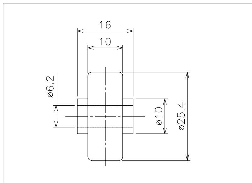
ホイル単品図
