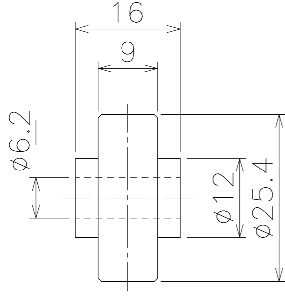
ホイール単品図
