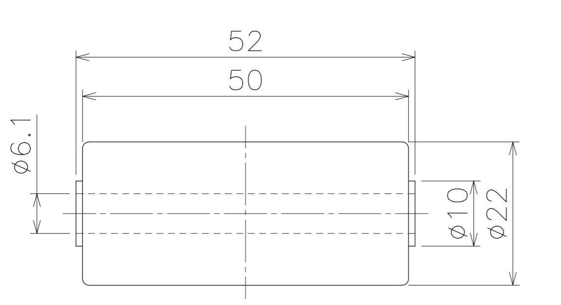
ホイール单品図
