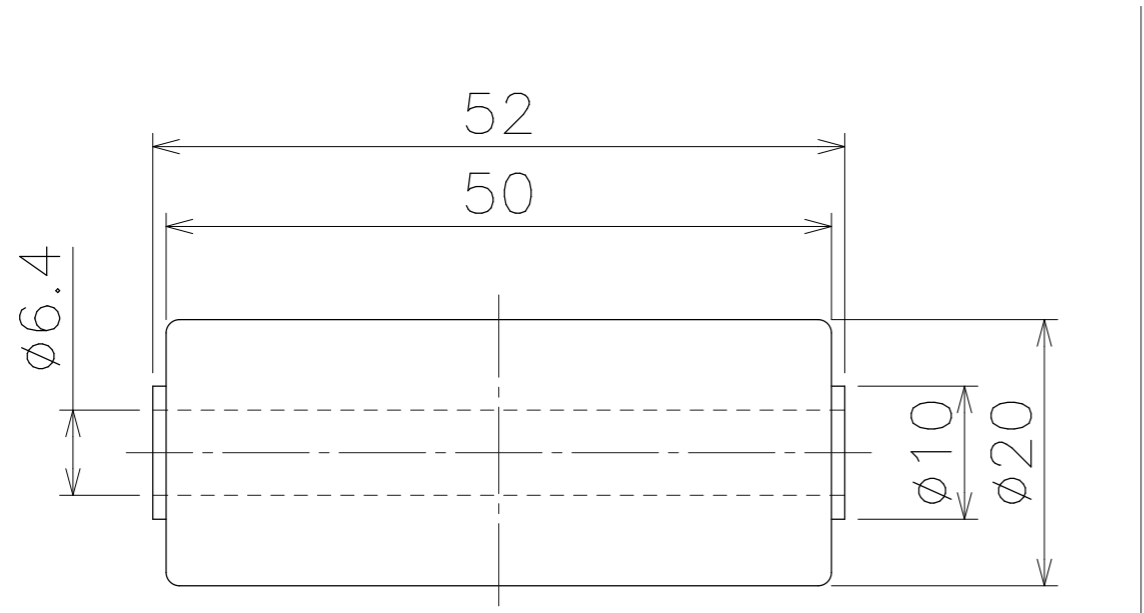
ホイール単品図
