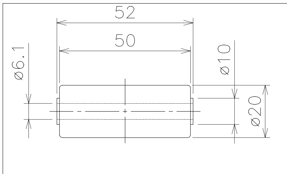
ホイール単品図
