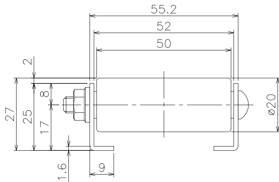
断面図
