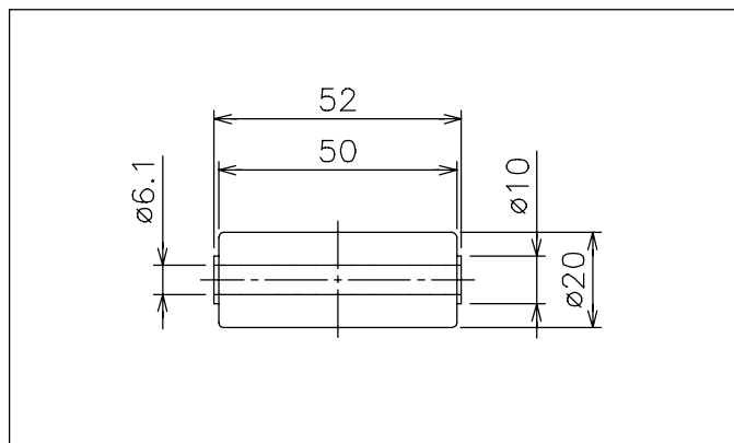
ホイル単品図
