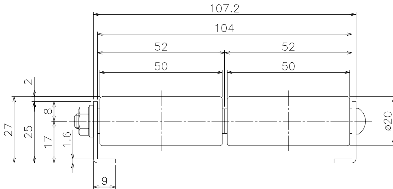
断面図
