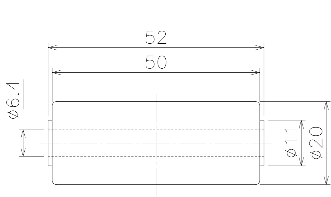
ホイール単品図
