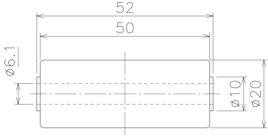
ホイール単品図
