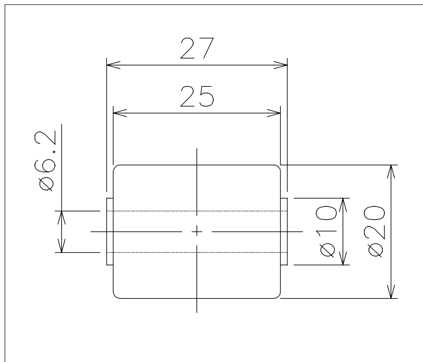
ホイール単品図
