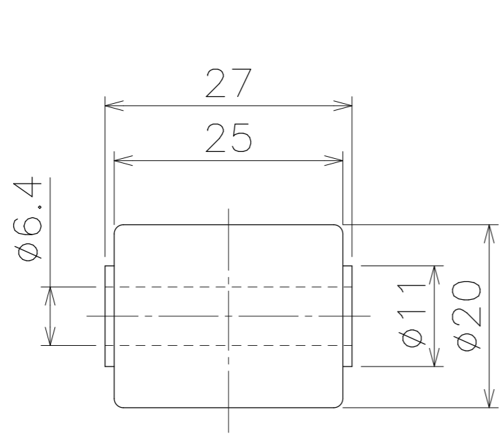
ホイール単品図
