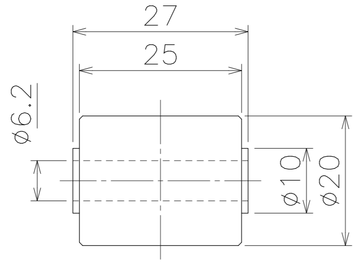
ホイール単品図
